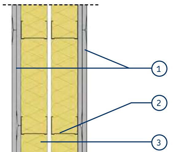
1. Lastre di gesso rivestito 2. Struttura in acciaio zincato
