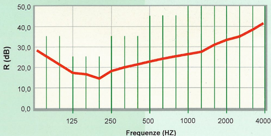
Potere fonoisolante R_w = 27,5 dB (certificazione CSI)
